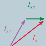
Fig 8 - Relation entre les courants résiduels de l'installation pour un réseau et des charges triphasées
