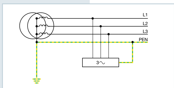
Fig.2 - Schéma TN-C
