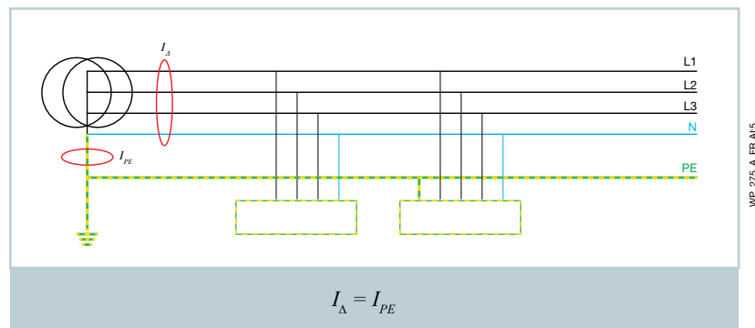
Fig 12 – Mesure du conducteur PE au général
