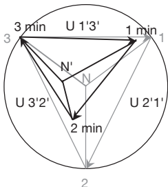
Réseau déséquilibré
