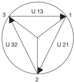
Réseau équilibré
