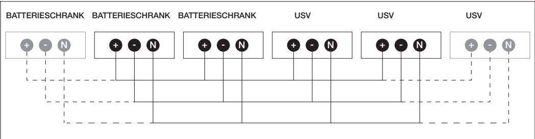
Anschlussbeispiel – verteilte Batterie
