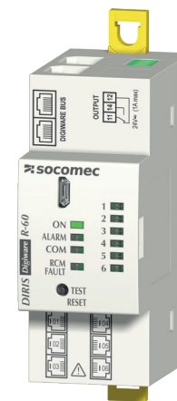
Dispositivo di monitoraggio della corrente residua DIRIS Digiware R-60 4829 0114
