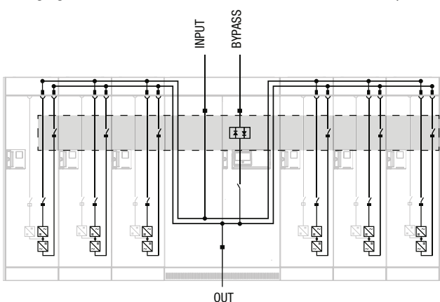
Architettura ibrida di bypass
