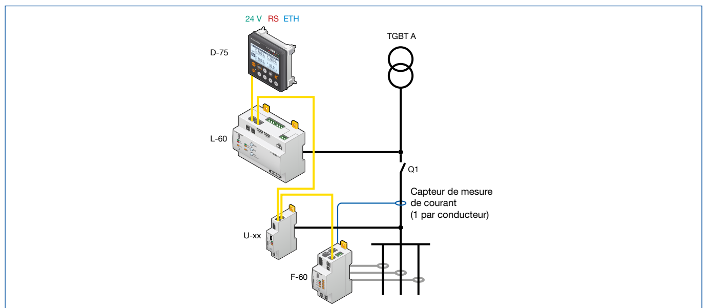
Fig. 3: Contrôle d'isolement + localisation de défauts + multi-mesure
