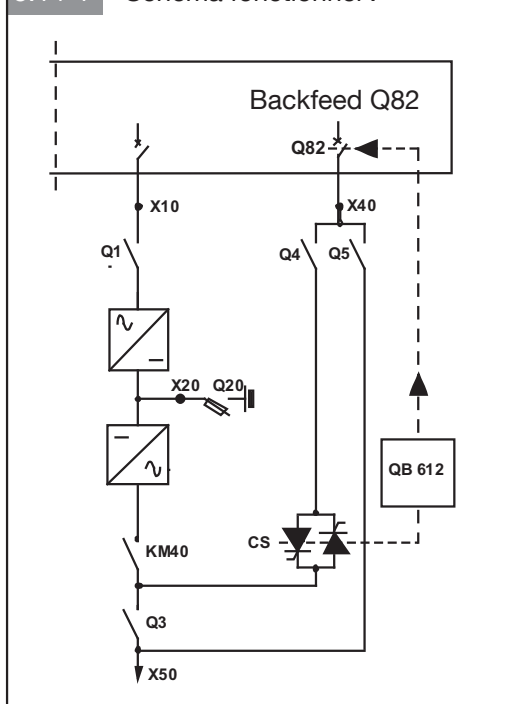
5.14-1 Schéma fonctionnel :
