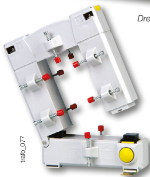
Teilbarer Stromwandler
