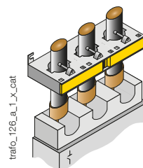
Dreiphasiger Stromwandler für Schienen- oder Kabeldurchführung
