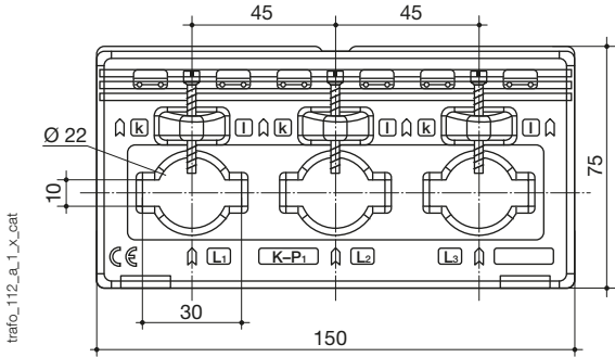
TCB3 22-30
