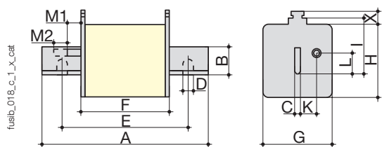
Dimensioni (mm) secondo la normativa IEC 60269-2-1
