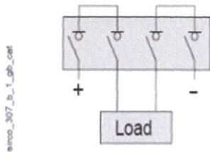
4 极 (1000VDC): 两极串联为正负极
